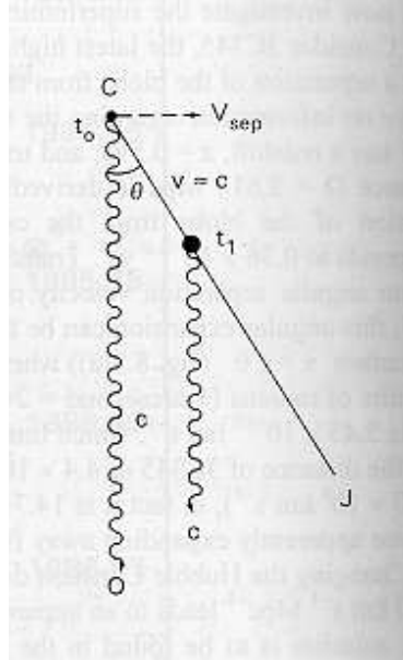
Abbildung 1.2: Schematische Darstellung des Projektionseffektes zur scheinbaren Überlichtgeschwindigkeit. Die Komponente bewegt sich schräg auf den Beobachter zu. Dadurch hat das zweite Signal einen kürzeren Laufweg. Der Beobachter sieht jedoch nur die Eigenbewegung senkrecht zur Sichtlinie und misst scheinbare Geschwindigkeiten, die grösser als die Lichtgeschwindigkeit sein können.
