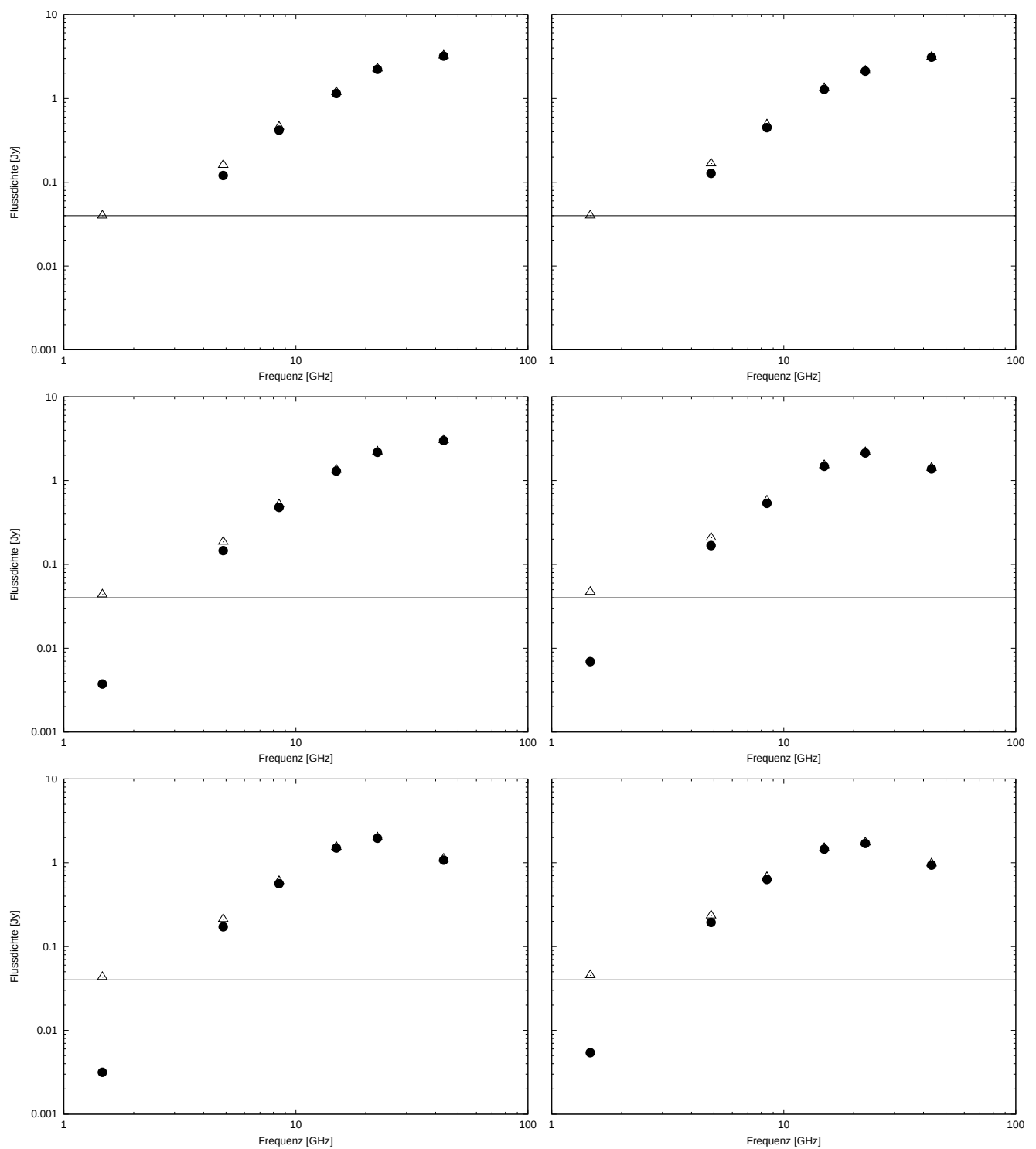
Abbildung 5.8: VLA-Spektrum vom 05.09.1998 (oben links), 01.10.1998 (oben rechts), 04.11.1998 (mitte links), 24.12.1998 (mitte rechts), 08.01.1999 (unten links) und 22.02.1999 (unten rechts). Der Peak ist zunächst konstant bei 43 GHz und fällt nach November 1998 schnell ab.
