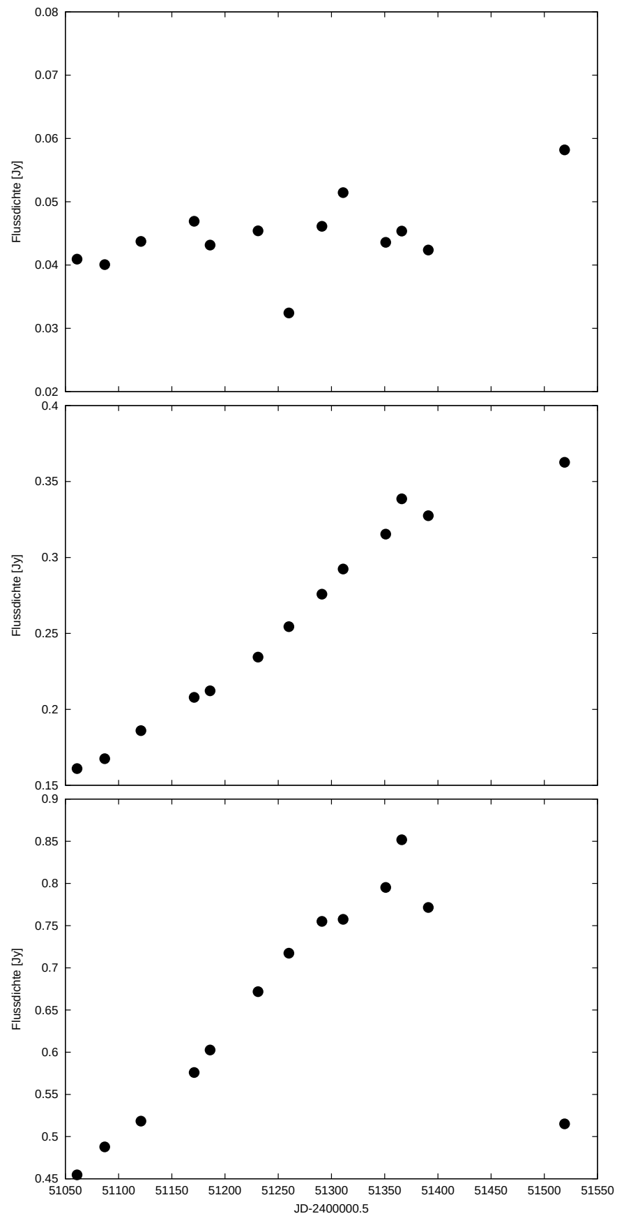
Abbildung 5.13: VLA-Lichtkurve bei 1.4 GHz (oben), 4.8 GHz (mitte) und 8.4 GHz (unten) des Radioausbruchs von III Zw 2.
