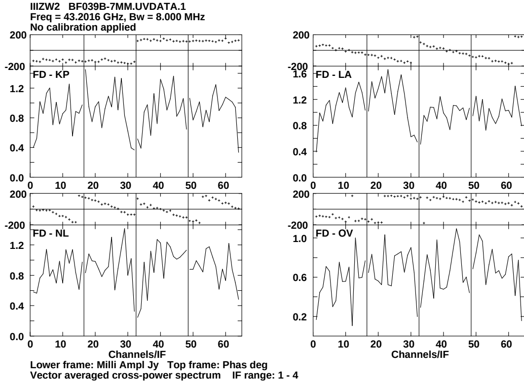
Abbildung 4.2: Ausgabe des Task POSSM für vier Basislinien. Die Einheiten der Amplitude sind noch willkürlich und die Phasen zeigen starke Variationen über die verschiedenen Kanäle.
