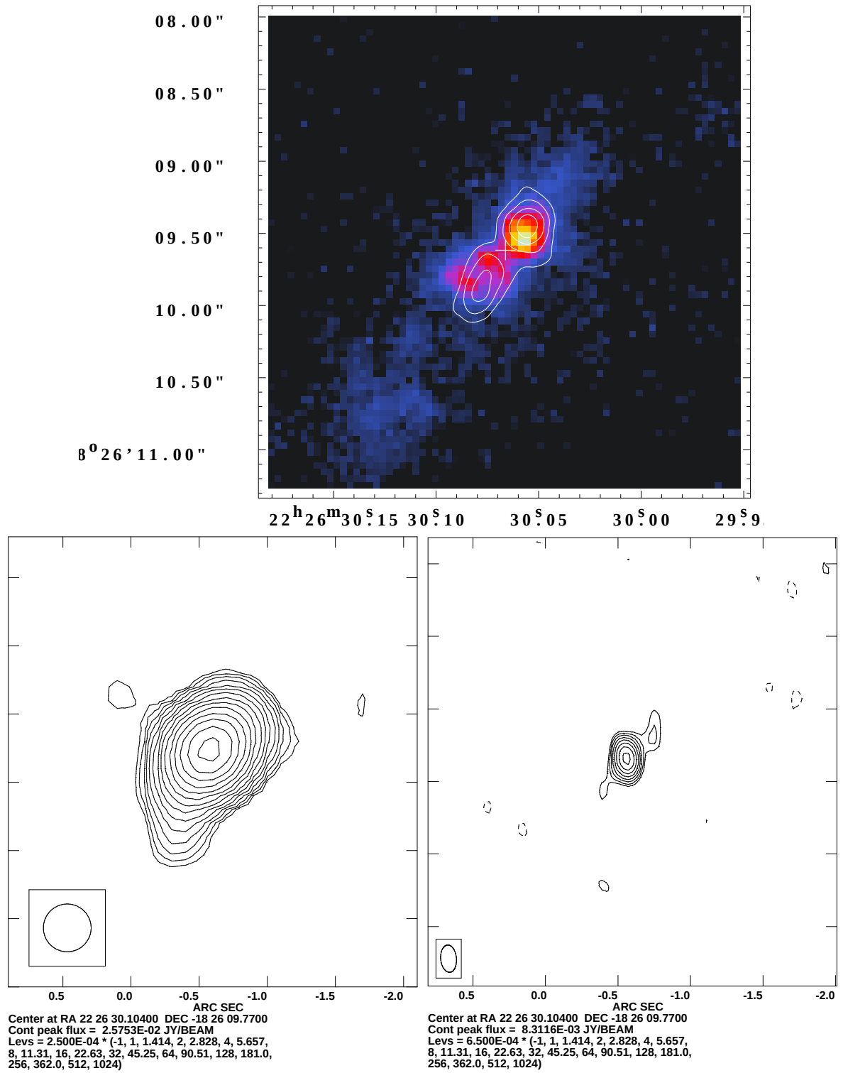
Abbildung A.1: TXS2226-184 bei 8.4 GHz (Konturen, oben) übergelegt mit einer HST H \alpha + [NII]-Karte. Bei der Radiokarte wurde der Kern entfernt um die ausgedehnte Struktur zu verdeutlichen. Zusätzlich sind Radiokarten bei 4.8 (links unten) und 15 GHz (rechts unten) gezeigt.
