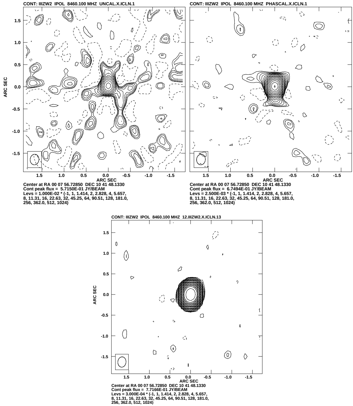
Abbildung 2.5: Karte von III Zw 2 bei 8.4 GHz mit dem VLA ohne Phasenkali- bration (oben links), nach reiner Phasenselbstkalibration (oben rechts) und nach Phasen- und Amplitu- denselbstkalibration (unten). Dabei ist zu beachten, dass die Konturniveaus jeweils um fast eine Grössenordnung gesunken sind.
