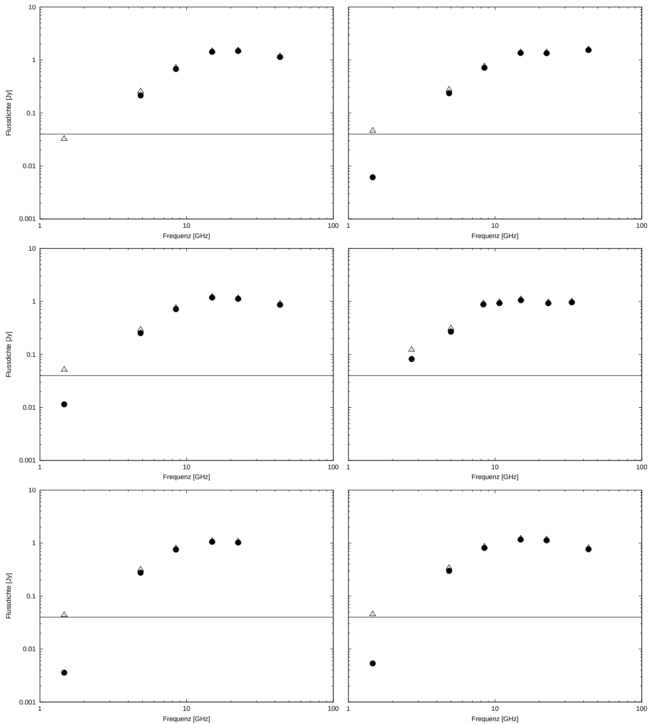
Abbildung 5.9: VLA-Spektrum vom 23.03.1999 (oben links), 23.04.1999 (oben rechts), 13.05.1999 (mitte links), das Effelsberg-Spektrum vom 08.06.1999 (mitte rechts), sowie die VLA-Spektren vom 22.06.1999 (unten links) und 07.07.1999 (unten rechts). Der Peak fällt zunächst auf 15 GHz und ändert sich danach nur noch langsam.
