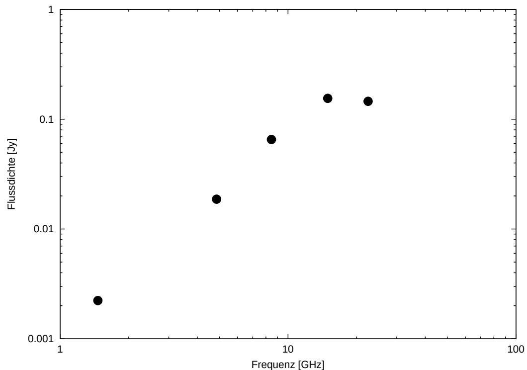
Abbildung 5.15: Spektrum des Ausbruchs vom Juli 1999.
