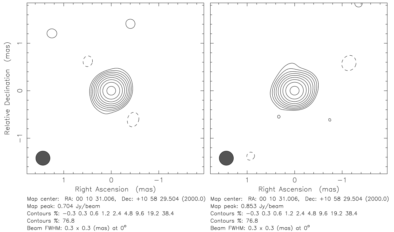
Abbildung 5.26: VLBA-Karte vom 16.02.1998 (links) und VLBA+Effelsberg Karte vom 13.06.1998 (rechts) von III Zw 2 bei 15 GHz rekonstruiert mit einem zirkularen 0.3 \times 0.3 mas Beam.
