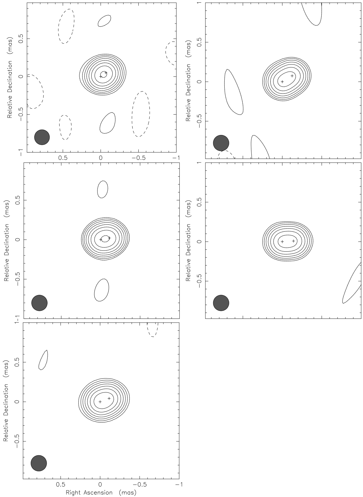
Abbildung 5.32: Modelle der 15 GHz-Daten. Die Kreuze stellen die Positionen der Komponenten dar. Es ist zu sehen, dass sich die Quelle während der ersten vier Epochen langsam ausdehnt. Zwischen der vierten und fünften Epoche fand keine weitere Expansion statt.
