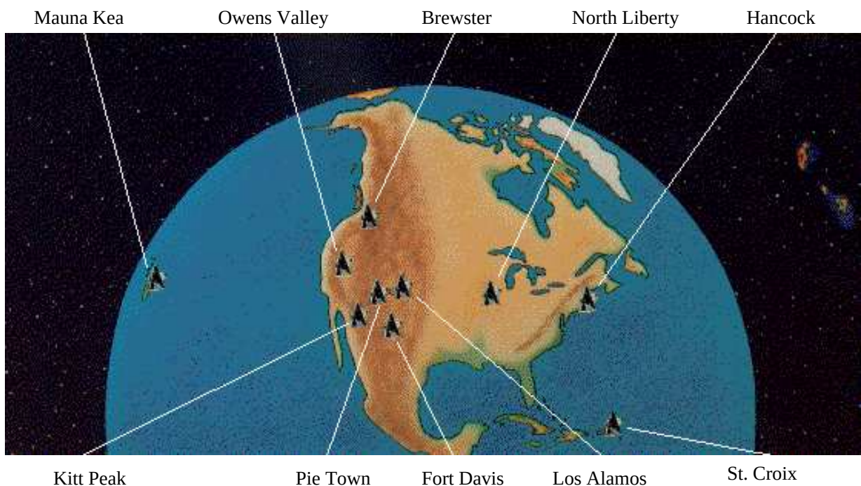
Abbildung 4.1: Positionen der 10 VLBA Antennen.
