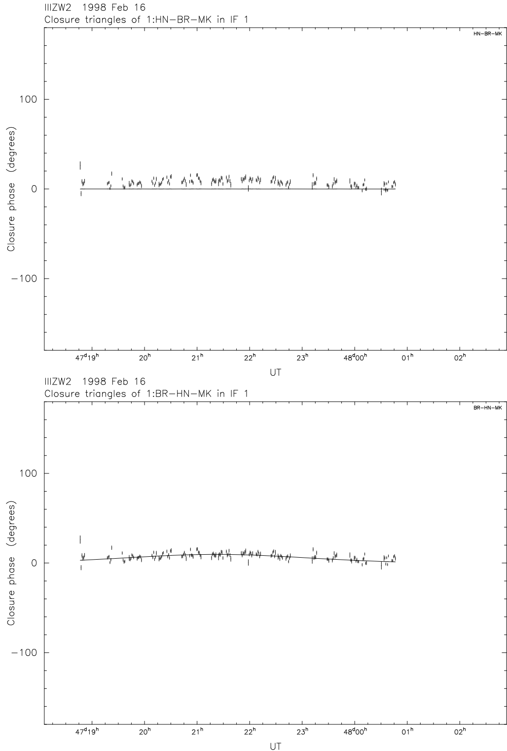
Abbildung 5.29: Closurephasen-Plot der Daten und des Modells (Linie) der ersten Epoche. Das obere Modell besteht aus nur einer Komponente und beschreibt die von Null verschiedene Closurephasen nur unzureichend. Das Modell aus zwei Komponenten stimmt jedoch sehr gut mit den Daten überein.
