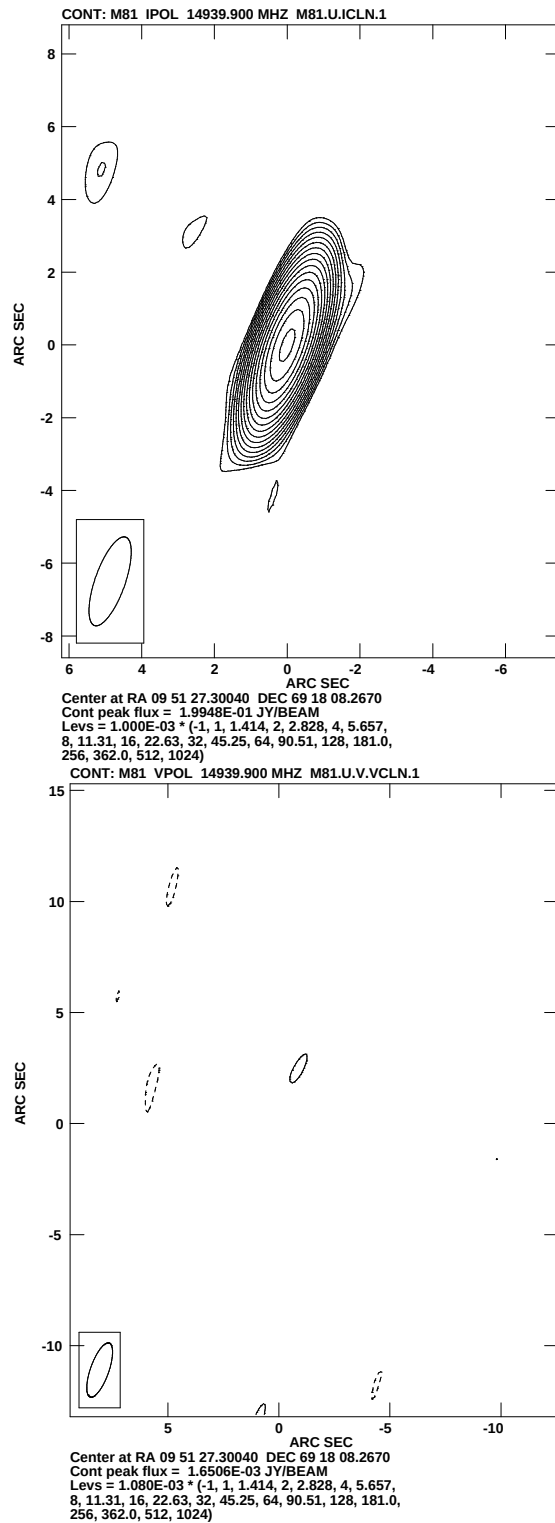
Abbildung A.4: M 81 in totaler Intensität bei 15 GHz (oben) und in zirkular polarisierter Strahlung (unten).
