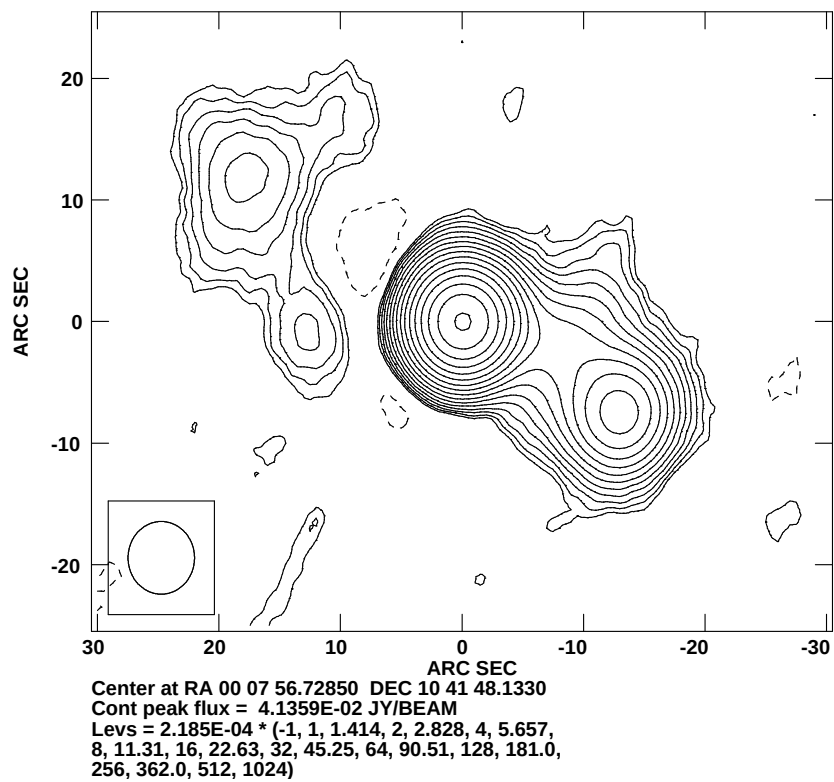
Abbildung 5.3: 1.4 GHz Karte von III Zw 2, zusammengesetzt aus 11 Epochen mit dem VLA in A, B, C und D-Konfiguration.
