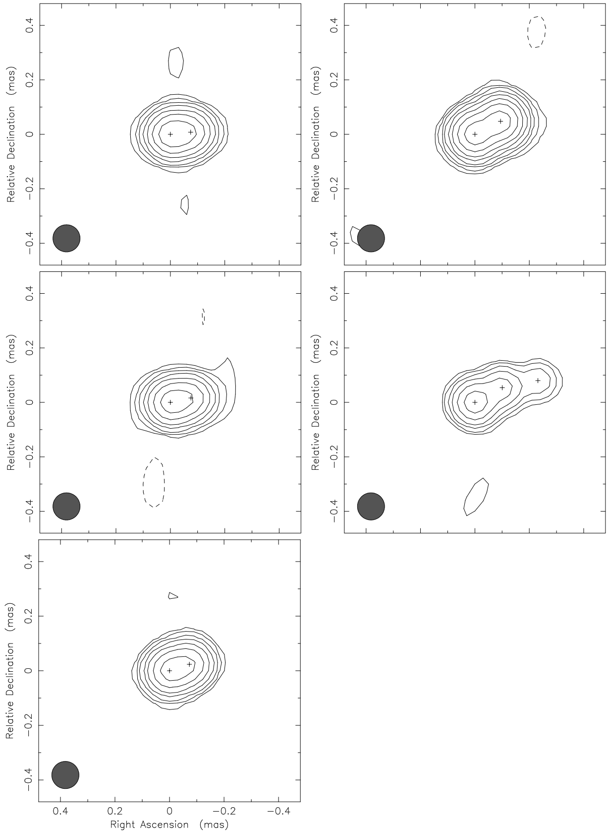
Abbildung 5.31: Modell-Komponenten der 43 GHz-Daten sowie die Residuen in den Karten. Die Kreuze stellen die Positionen der Komponenten dar. Es ist deutlich zu sehen, dass sich die ersten drei Epochen kaum voneinander unterscheiden (linke Spalte), während danach eine schnelle Expansion einsetzte (rechte Spalte).
