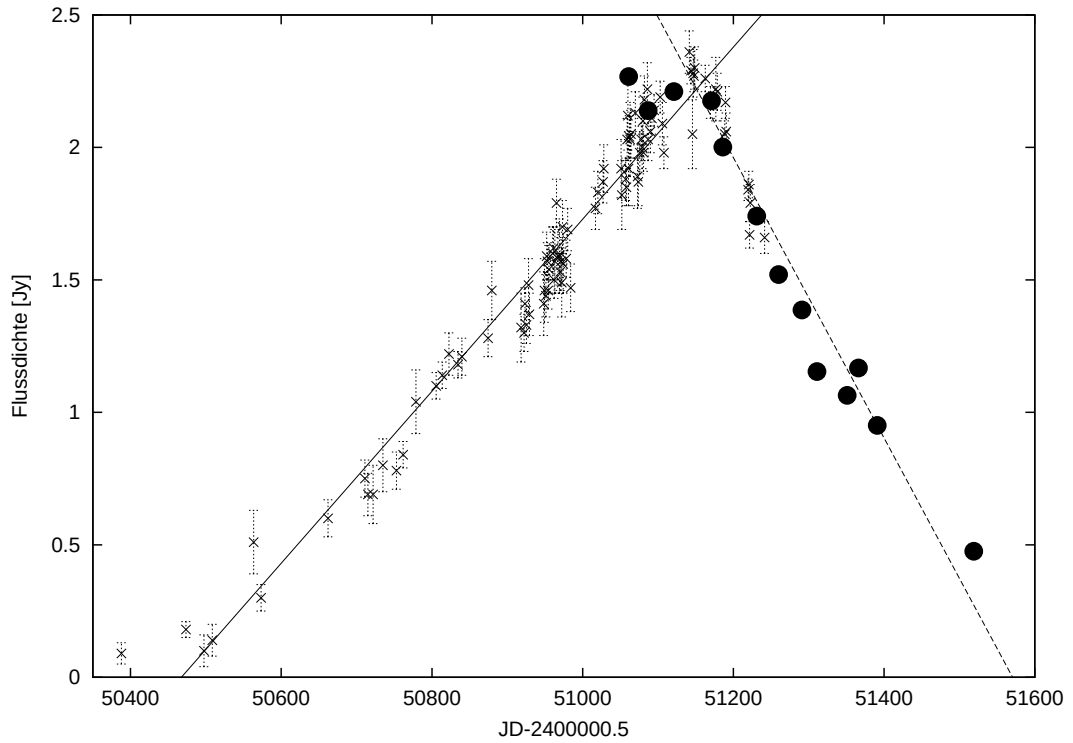
Abbildung 5.12: 22 GHz-Lichtkurve des Radioausbruchs von III Zw 2. Die schwarzen Kreise sind die VLA-Messdaten.
