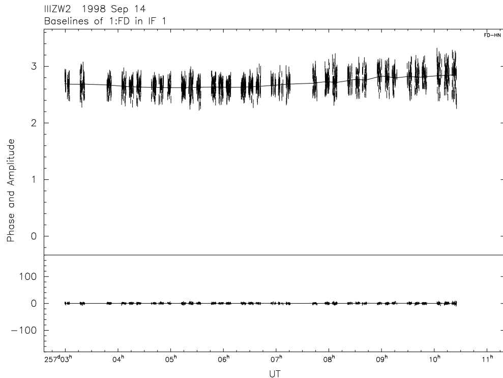
Abbildung 4.4: Zeitliche Entwicklung der Amplitude und der Phase für die Basislinie Fort Davis - Hancock. Die durchgezogene Linie stellt das aktuelle Modell dar. Es ist zu sehen, das Modell und Daten sehr gut übereinstimmen.
