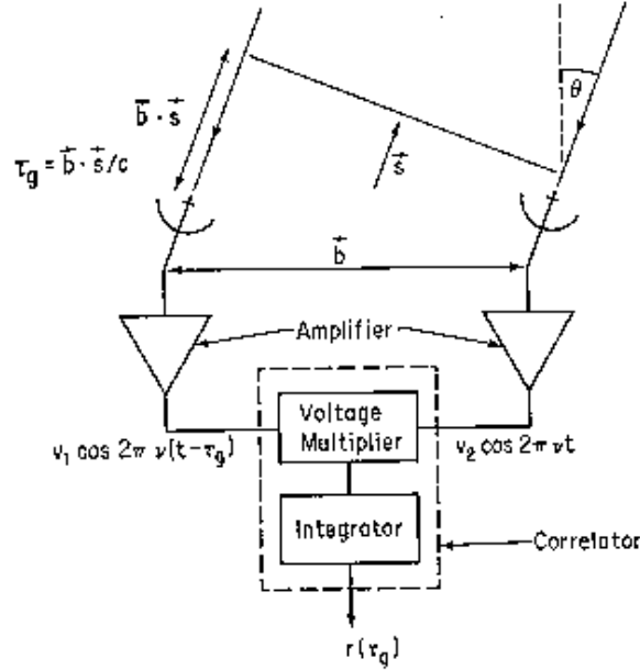
Abbildung 2.3: Schematische Darstellung eines Zwei-Element Interferometers (entnommen aus Thompson 1999).
