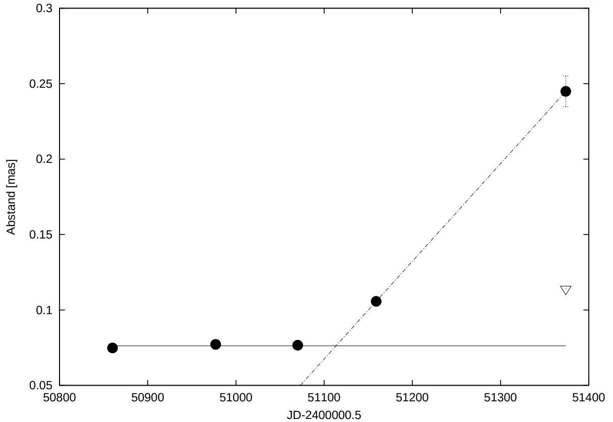
Abbildung 6.1: Abstand der äusseren Komponenten (Punkte) bei 43 GHz. Während die ersten drei Epochen mit einer Expansionsgeschwindigkeit von \leq 0.04 c (durchgezogene Linie) verträglich sind, gab es zwischen der vierten und fünften Epoche eine Expansion mit 1.25 c (gestrichelte Linie). Zusätzlich ist noch der Abstand der beiden inneren Komponenten der fünften Epoche gezeigt (Dreieck).
