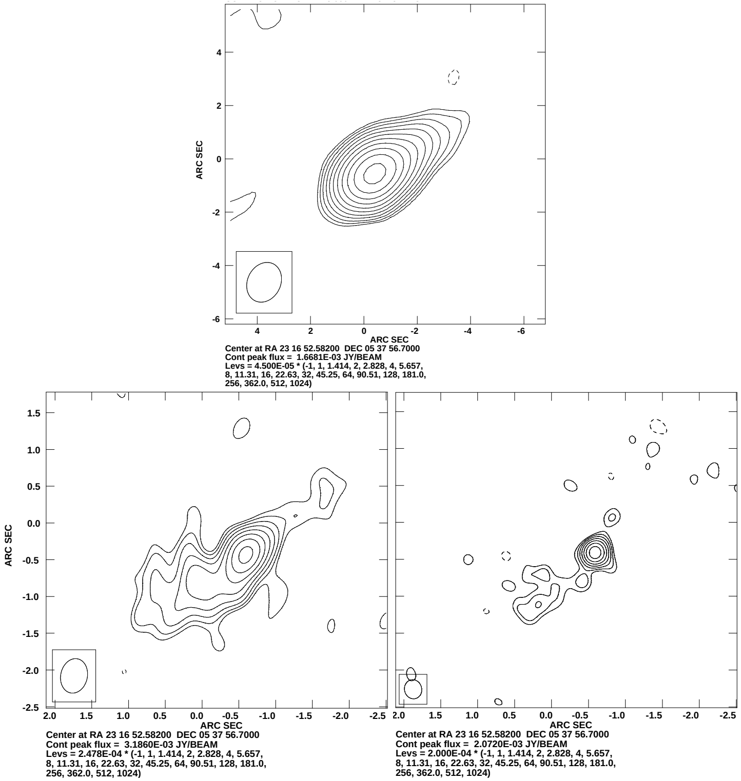
Abbildung A.2: IC 1481 bei 1.4 (oben), 4.8 (links unten) und 8.4 GHz (rechts unten).
