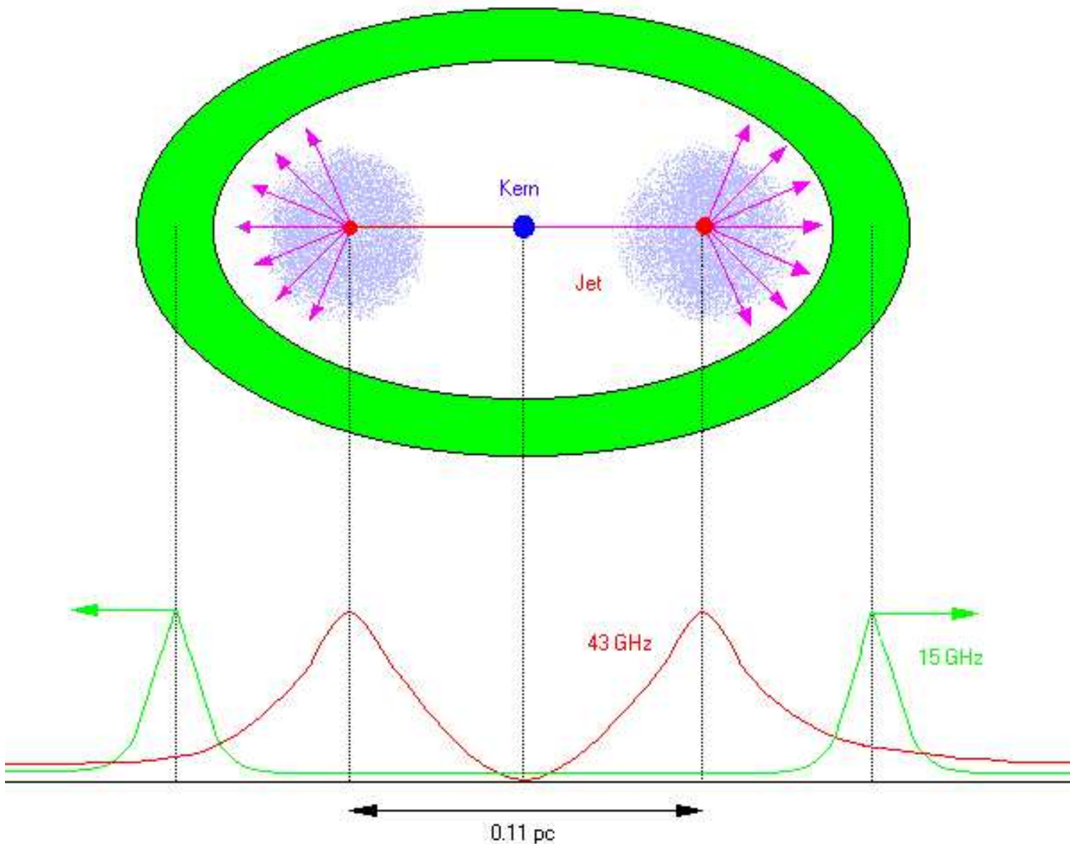
Abbildung 6.4: Das “Luftballon-Modell”. Hier ist ein doppelseitiger Jet zu sehen, der in einem Hinderniss einen Schock ausbildet (rot). Das post-Schock Material expandiert mit Schallgeschwindigkeit (violette Pfeile). Die beiden Kurven repräsentieren einen Schnitt durch die Quelle bei 43 und 15 GHz. Bei 43 GHz (rote Kurve) ist die Quelle optisch dünn, so dass man die beiden stationären Schocks sieht, während bei 15 GHz die Quelle optisch dick ist und man nur auf die \tau \approx 1 -Fläche (grün) sieht, die mit Schallgeschwindigkeit expandiert.
