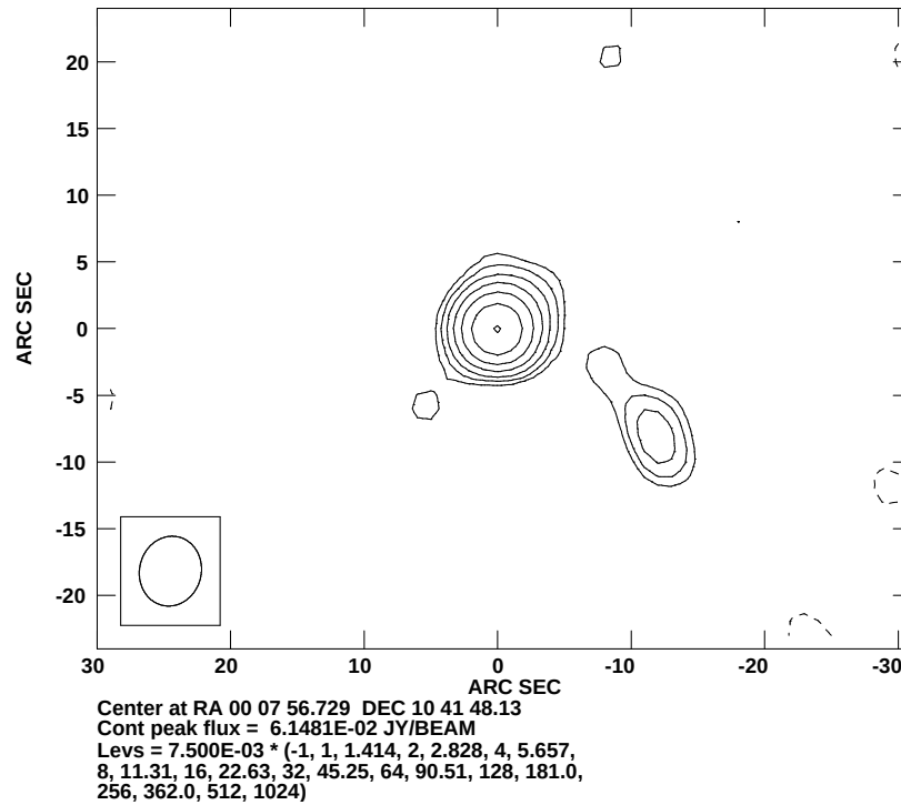
Abbildung 5.2: III Zw 2 bei 350 MHz. Zu erkennen ist der Kern und der helle Hotspot. Die jetförmige Verbindung ist nur angedeutet.
