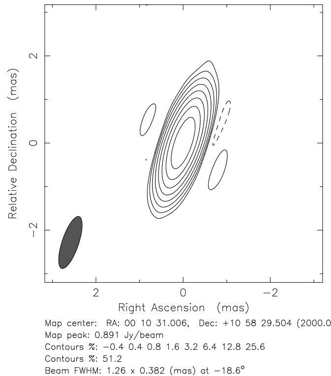
Abbildung 5.25: VLBA-Karte vom 15.07.1999 von III Zw 2 bei 15 GHz rekonstruiert mit dem Originalbeam.
