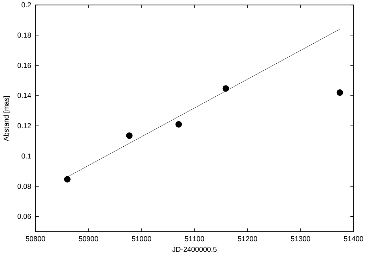
Abbildung 6.3: Abstand der Komponenten bei 15 GHz. Während die ersten vier Epochen eine Expansionsgeschwindigkeit von 0.6 c (durchgezogene Linie) zeigen, gab es zwischen der vierten und fünften Epoche keine weitere Expansion.
