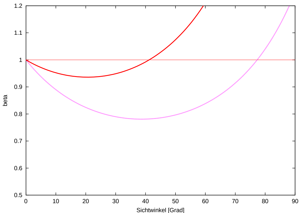
Abbildung 6.2: Reale Geschwindigkeit \beta in Abhängigkeit vom Blickwinkel für die beiden Werte 1.25 c (untere gepunktete Linie) und 2.66 c (obere durchgezogene Linie) für die scheinbare Überlichtgeschwindigkeit. Da \beta < 1 sein muss, ergibt dies den maximalen Blickwinkel von 78° bzw. 41°.
