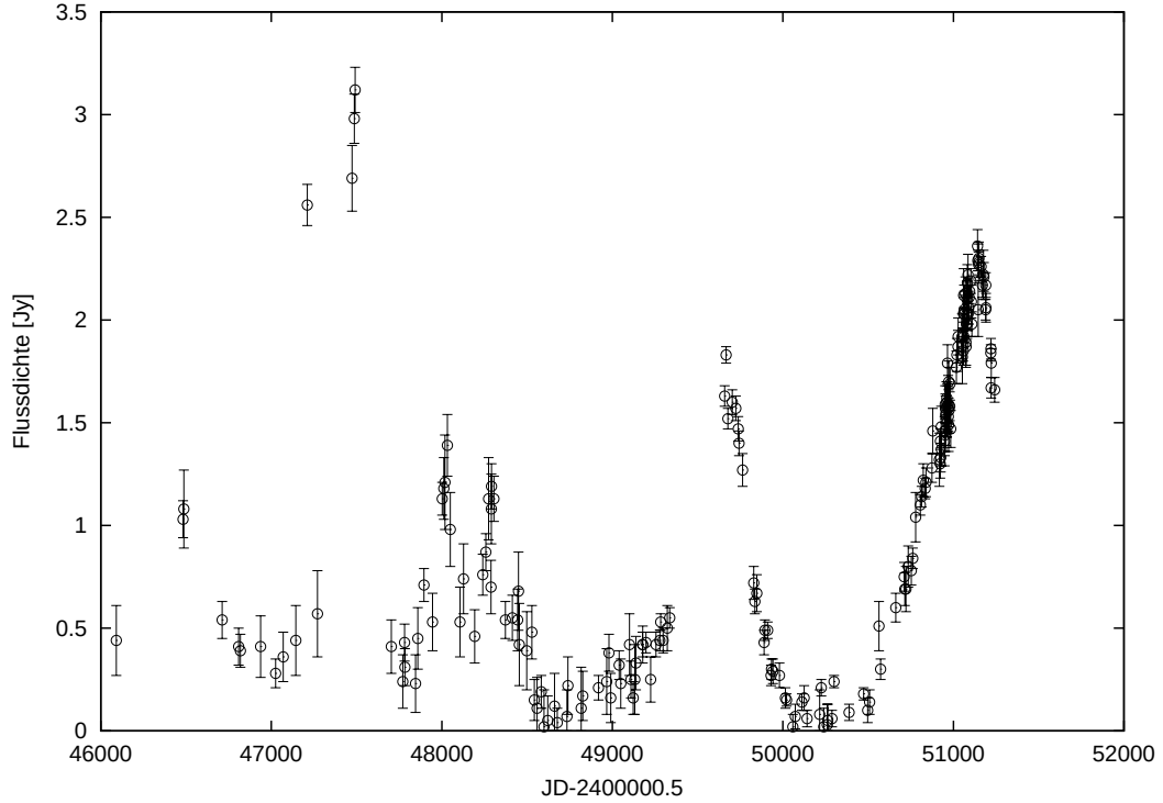
Abbildung 1.4: Langzeitlichtkurve bei 22 GHz von III Zw 2 von 1985 bis 1999 aufgenommen mit dem Metsähovi Radio Observatory in Kylmäälä, Finnland. Der letzte Ausbruch startete im Frühsommer 1997 und erreichte seinen Höhepunkt bei 22 GHz im November 1998 (H. Teräsanta, persönliche Mitteilung).
