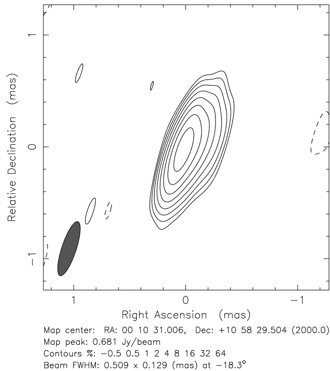
Abbildung 5.19: VLBA-Karte vom 15.07.1999 von III Zw 2 bei 43 GHz rekonstruiert mit dem Originalbeam. Es ist deutlich zu sehen, dass der Kern nach Nordwesten ausgedehnt ist.
