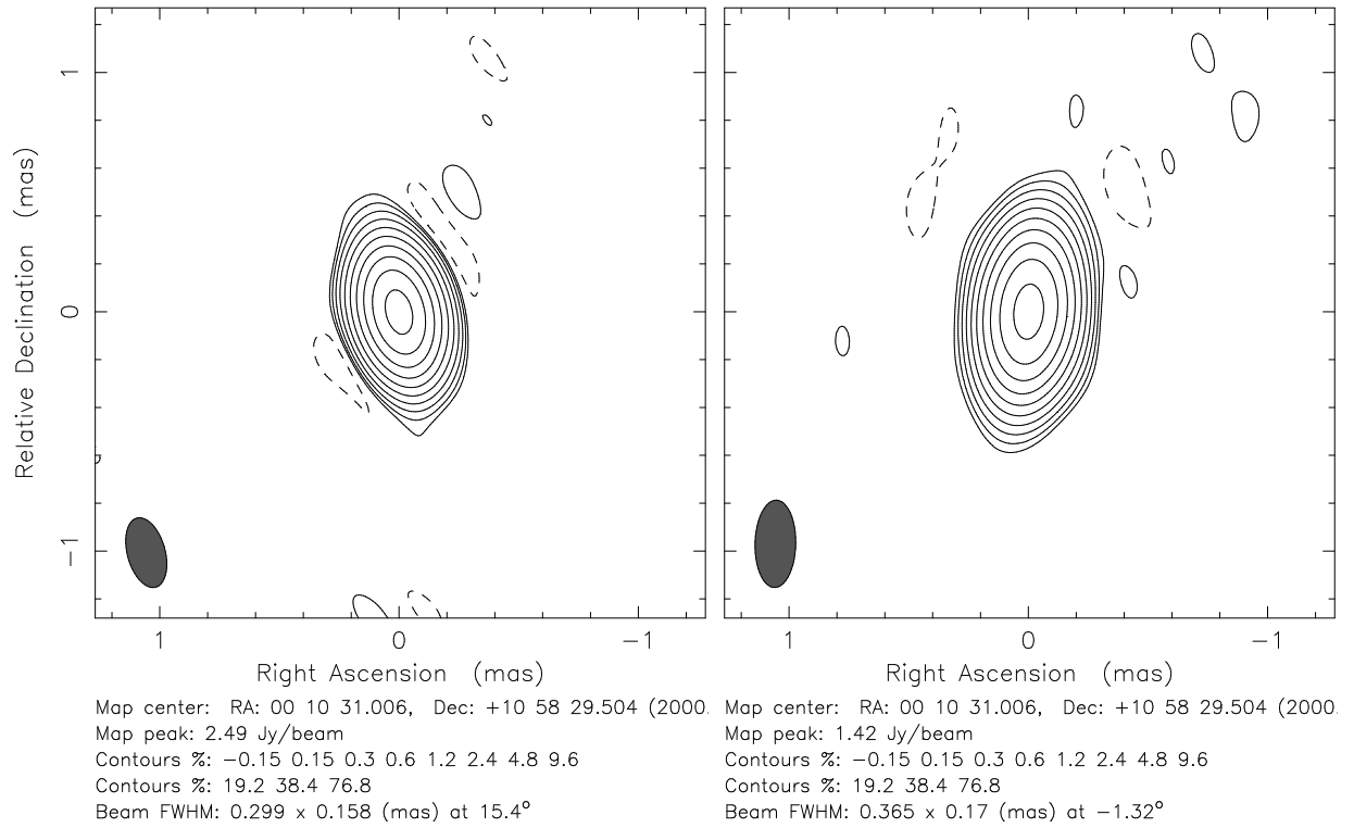
Abbildung 5.17: VLBA-Karte vom 16.02.1998 (links) und VLBA+Effelsberg Karte vom 13.06.1998 (rechts) von III Zw 2 bei 43 GHz rekonstruiert mit dem Originalbeam.
