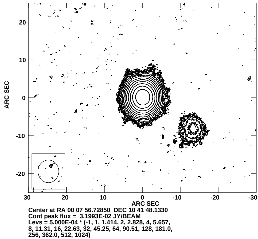
Abbildung 5.6: 15 GHz Karte von III Zw 2, zusammengesetzt aus 11 Epochen mit dem VLA in A, B, C und D-Konfiguration.
