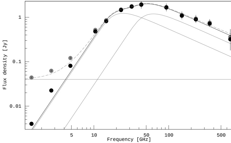
Abbildung 1.5: Breitbandspektrum von III Zw 2 vom Mai 1998. Die grauen Punkte zeigen die gemessenen Flussdichten an, während die schwarzen Punkten, bei denen der Fluss vor dem Ausbruch von 40 mJy abgezogen wurde, das Spektrum des Ausbruchs anzeigt. Zusätzlich sind noch die beiden angepassten Synchrotronkomponenten, der 40 mJy Level und ihre Summe angezeigt (entnommen aus Falcke et al. 1999).
