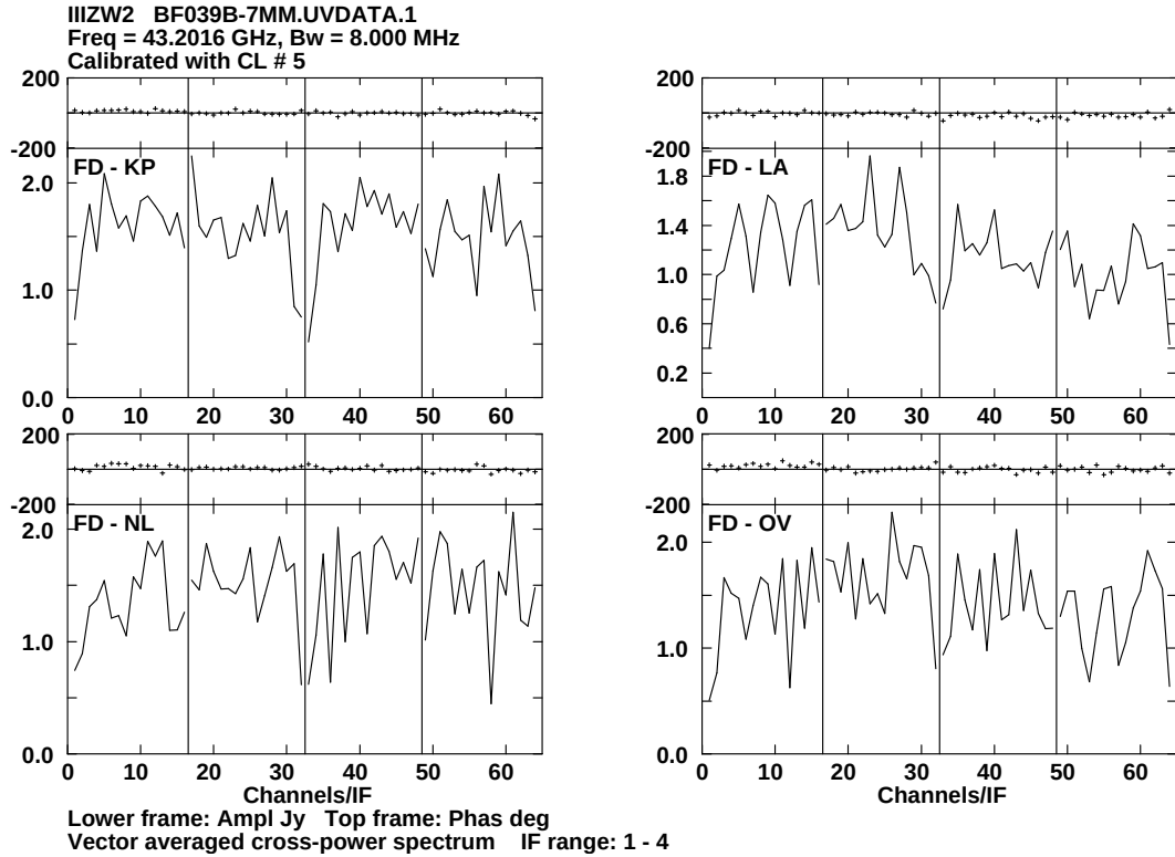
Abbildung 4.3: Daten nach der Kalibration. Die Einheit der Amplituden ist nun in Jansky angegeben und die Phasen sind einheitlich.
