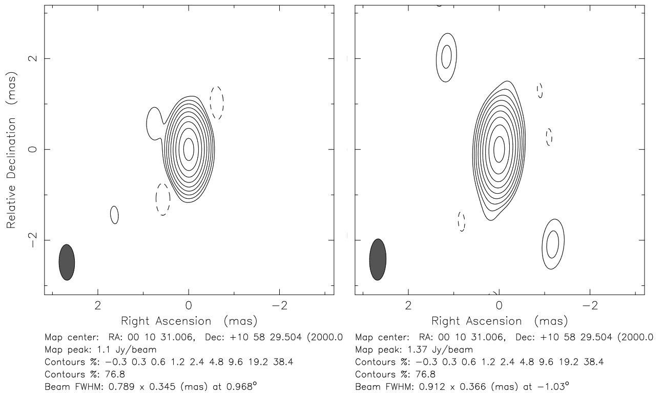
Abbildung 5.24: VLBA-Karte vom 14.09.1998 (links) und vom 12.12.1998 (rechts) von III Zw 2 bei 15 GHz rekonstruiert mit dem Originalbeam.
