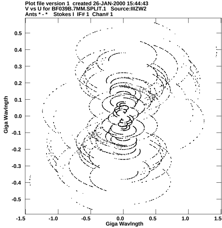
Abbildung 2.2: UV-Abdeckung der Beobachtung vom 13.06.1998 mit dem VLBA und Effelsberg. Die Dauer der Beobachtung betrug 8 Stunden. Die einzelnen Spuren gehören jeweils zu einer Basislinie und zeigen die Drehung der Erde im Raum.
