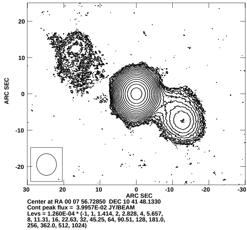
Abbildung 5.5: 8.4 GHz Karte von III Zw 2, zusammengesetzt aus 11 Epochen mit dem VLA in A, B, C und D-Konfiguration.
