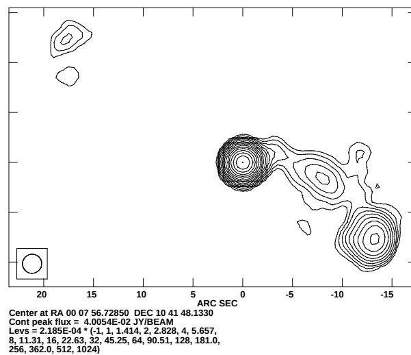
Abbildung 5.1: 1.4 GHz Karte von III Zw 2. Die Karte ist eine Kombination von 11 Epochen. Die Beamgrösse beträgt 1.93 \times 1.91 Bogensekunden bei einem Positionswinkel (P.A.) von -55.48^\circ . Die uv-Abdeckung dieser Karte war in Abbildung 3.3 zu sehen.
