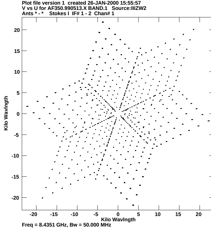
Abbildung 2.1: UV-Abdeckung einer 4 Minuten Beobachtung vom 13.05.1999 mit dem VLA. Die Y-Struktur des VLA ist deutlich zu erkennen. Wegen der Hermitizität ist jeder Messpunkt nochmal am Ursprung gespiegelt zu erkennen.
