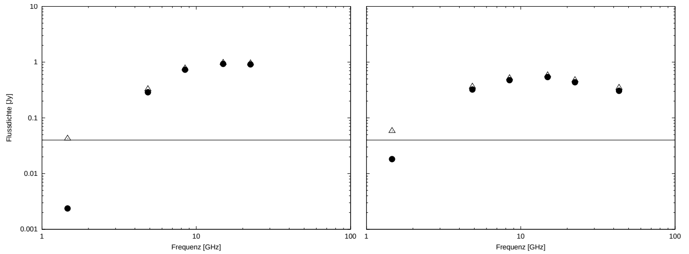
Abbildung 5.10: VLA-Spektrum vom 01.08.1999 (links) und vom 25.01.2000 (rechts).
