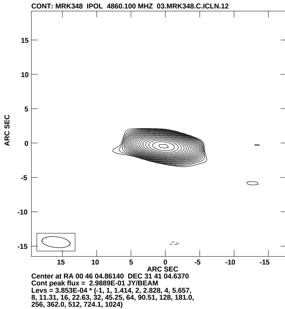
Abbildung A.3: Mrk 348 bei 4.8 GHz vom 04.11.1998.
