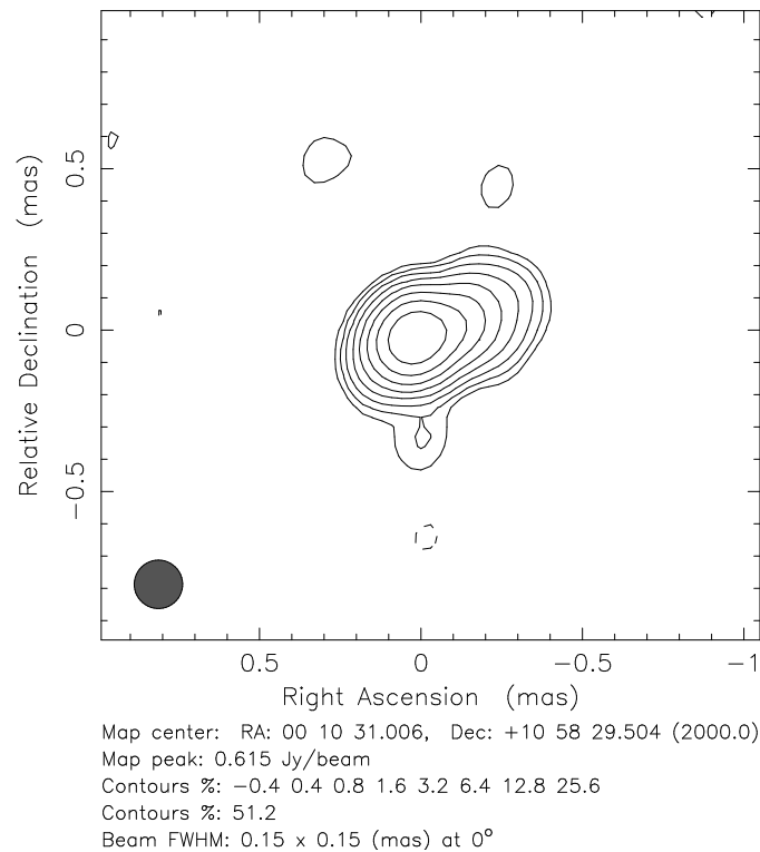
Abbildung 5.22: VLBA-Karte vom 15.07.1999 von III Zw 2 bei 43 GHz rekonstruiert mit einem zirkularen 0.15 \times 0.15 mas Beam. Es ist deutlich zu sehen, dass der Kern nach Nordwesten ausgedehnt ist.
