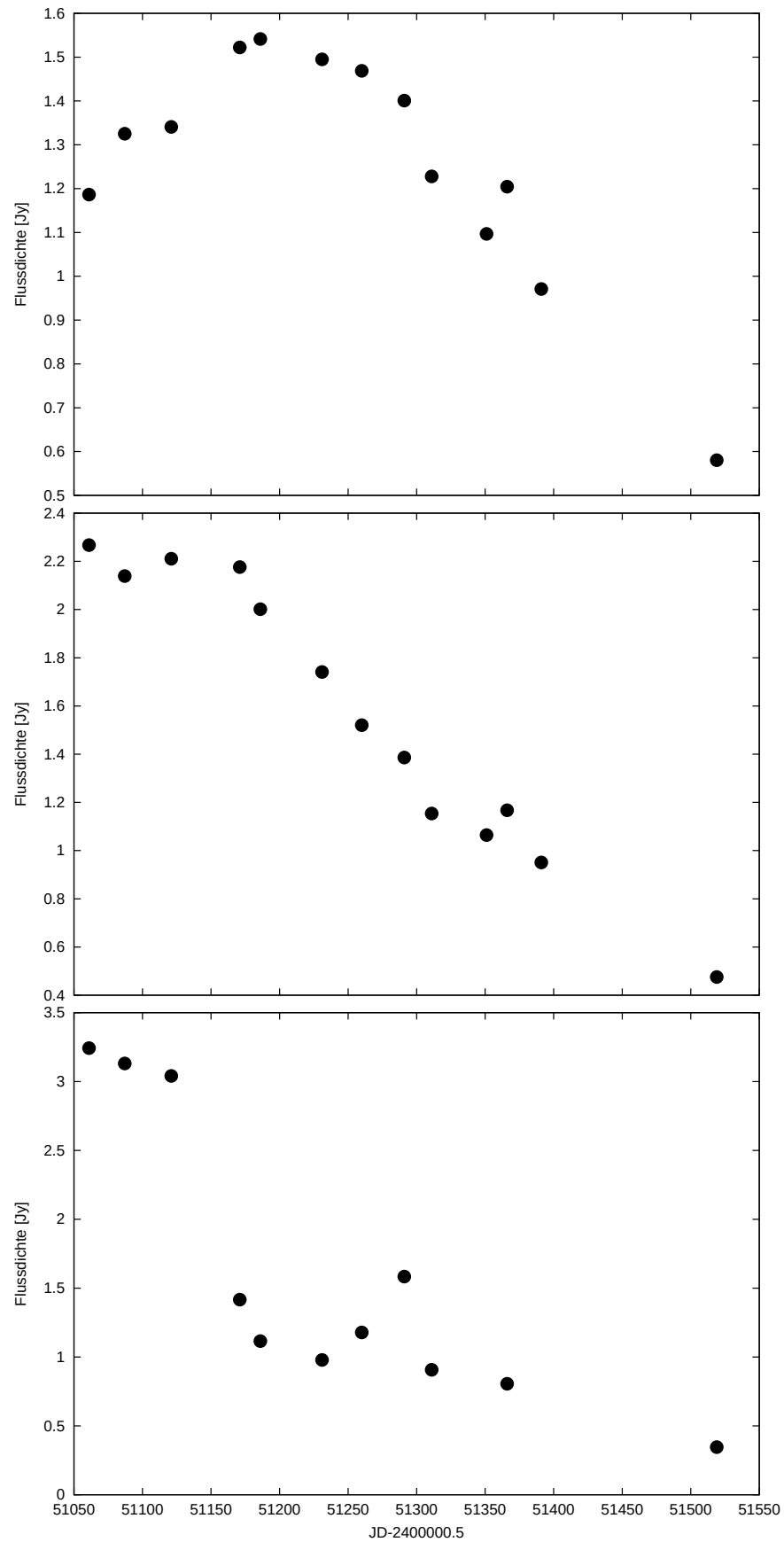
Abbildung 5.14: VLA-Lichtkurve bei 15 GHz (oben), 22 GHz (mitte) und 43 GHz (unten) des Radioausbruchs von III Zw 2.
