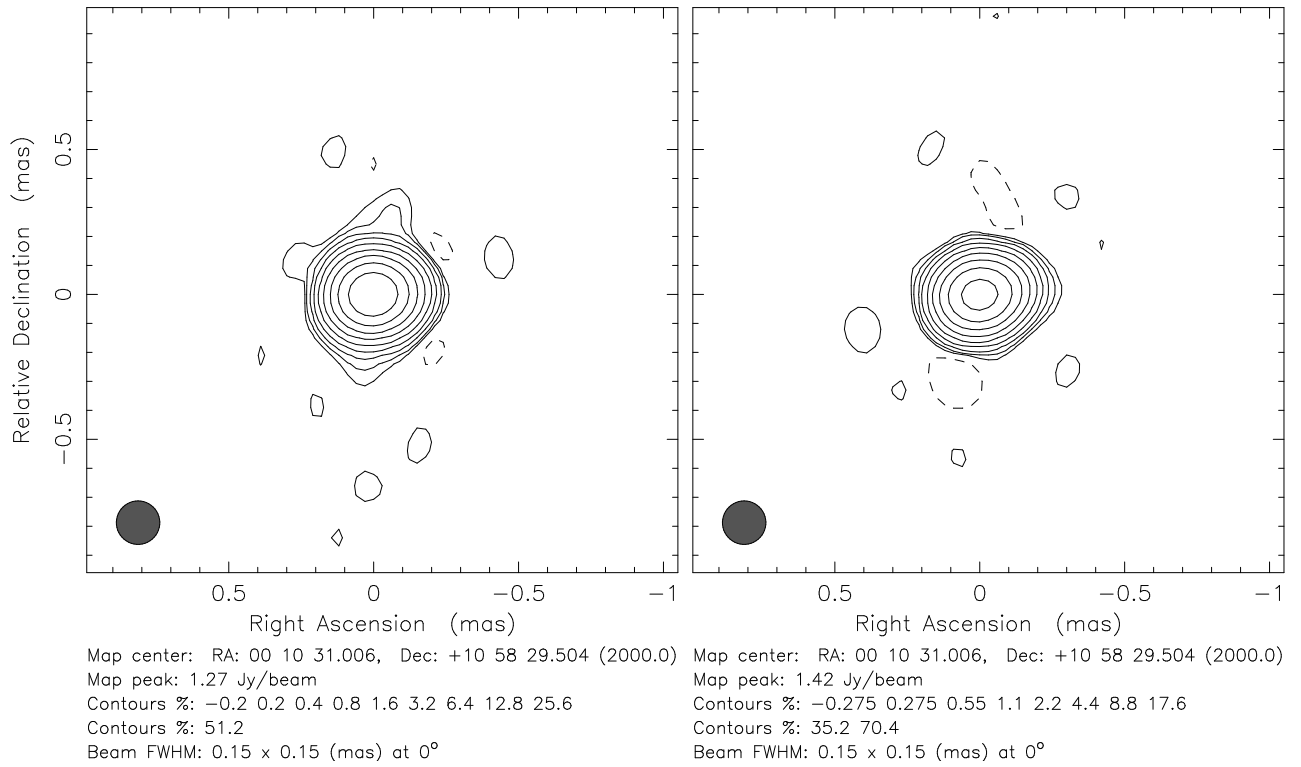
Abbildung 5.20: VLBA-Karte vom 16.02.1998 (links) und VLBA+Effelsberg Karte vom 13.06.1998 (rechts) von III Zw 2 bei 43 GHz rekonstruiert mit einem zirkularen 0.15 \times 0.15 mas Beam.
