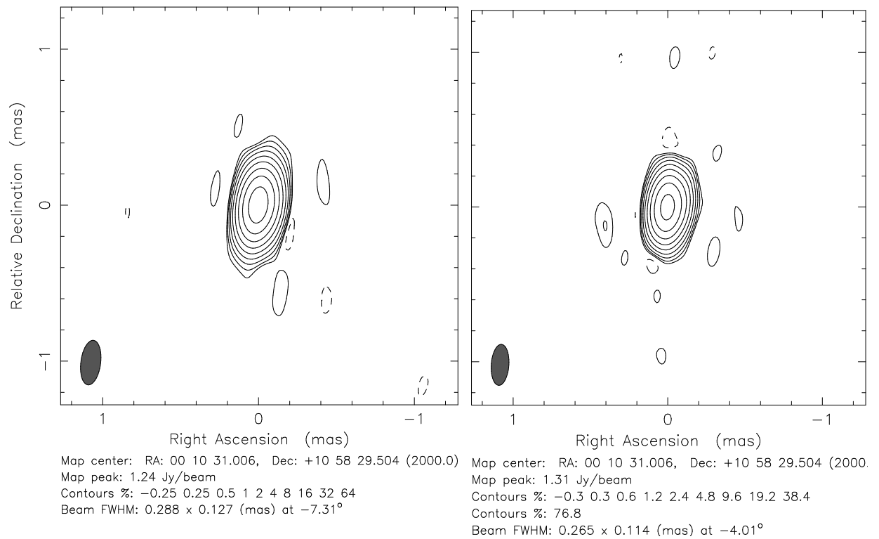
Abbildung 5.18: VLBA-Karte vom 14.09.1998 (links) und vom 12.12.1998 (rechts) von III Zw 2 bei 43 GHz rekonstruiert mit dem Originalbeam.
