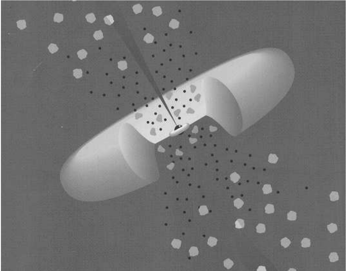
Abbildung 1.1: Schematische Darstellung des Kernbereichs einer aktiven Galaxie. Im Zentrum liegt das schwarze Loch, welches von einer Akkretionsscheibe umgeben wird. Die Wolken in der Nähe des Zentrum symbolisieren die BLR, während die äusseren Wolken die NLR darstellen. Das Zentrum ist von einem absorbierenden Staubtorus (hier aufgeschnitten) umgeben. Zusätzlich schiesst noch ein doppelseitiger Jet von der Innenseite der Akkretionsscheibe senkrecht zu dieser nach aussen. Der Counter-Jet ist nur sehr schwach angedeutet und nur zu erahnen. (entnommen aus Krolik 1999).
