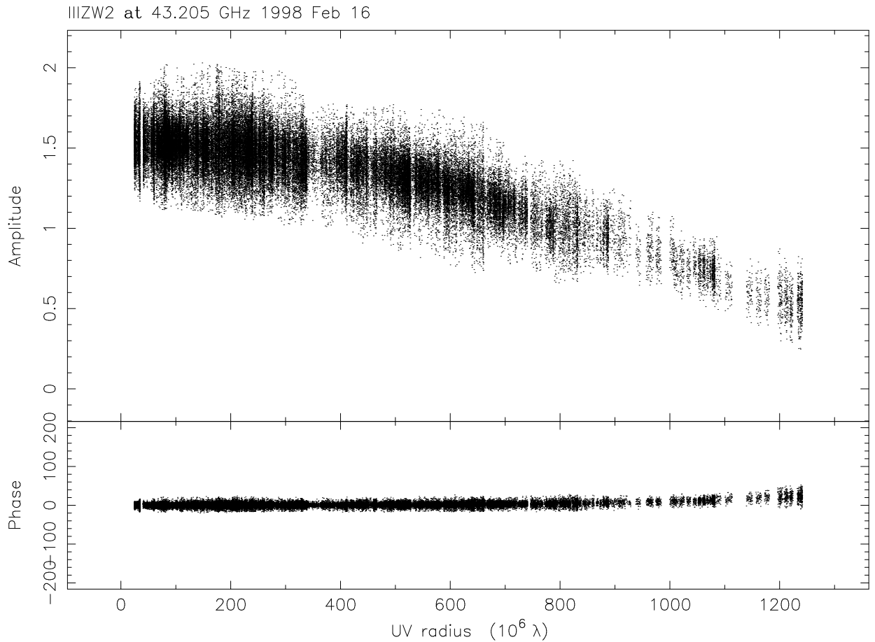
Abbildung 5.16: Visibilities gegen die Länge der Basislinie. Die Amplitude fällt deutlich auf etwa ein Drittel bei 1200M\lambda . Dies ist typisch für eine aufgelöste Struktur.
