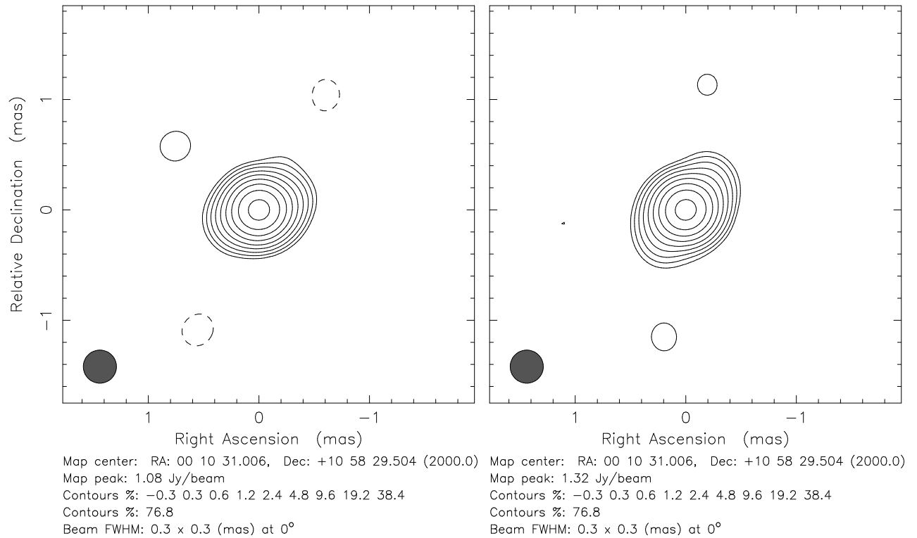
Abbildung 5.27: VLBA-Karte vom 14.09.1998 (links) und vom 12.12.1998 (rechts) von III Zw 2 bei 15 GHz rekonstruiert mit einem zirkularen 0.3 \times 0.3 mas Beam.
