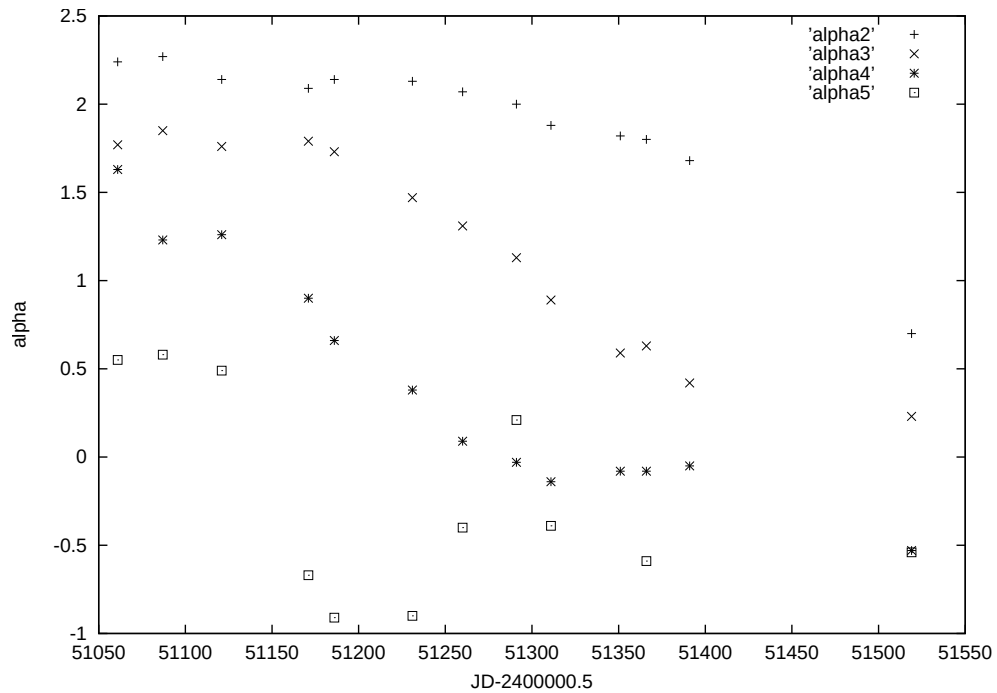
Abbildung 5.11: Zeitliche Entwicklung der Spektralindices. Hierbei stehen alpha2, alpha3, alpha4 und alpha5 für die \alpha_{4.8-8.4} , \alpha_{8.4-15} , \alpha_{14-22} und \alpha_{22-43} aus Tabelle 5.3. Es ist zu sehen, dass der Spektralindex für höhere Frequenzen schneller abfällt als bei niedrigen. Bei \alpha_{22-43} ist ein starkes Springen der Werte zu sehen, was mit der Ungenauigkeit bei der Bestimmung der 43 GHz Flussdichte zu erklären ist.
