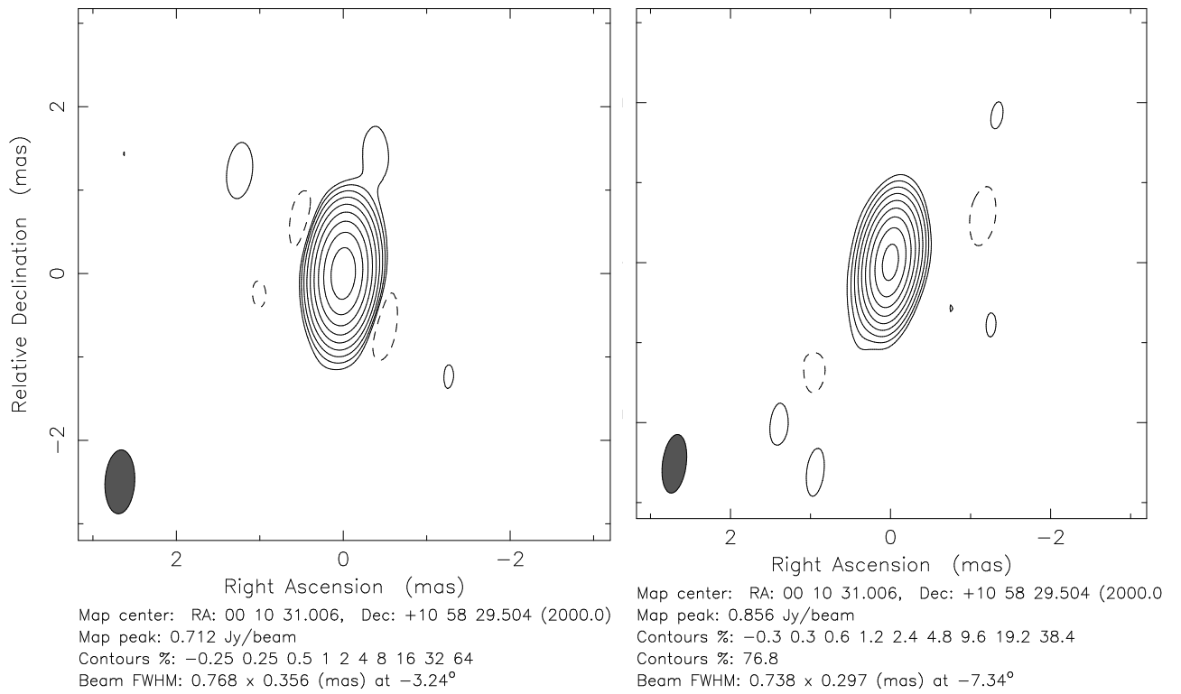
Abbildung 5.23: VLBA-Karte vom 16.02.1998 (links) und VLBA+Effelsberg Karte vom 13.06.1998 (rechts) von III Zw 2 bei 15 GHz rekonstruiert mit dem Originalbeam.
