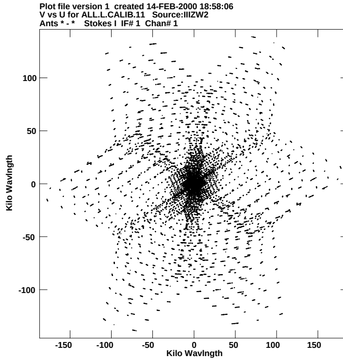
Abbildung 3.3: uv-Abdeckung des kombinierten Datensatz aus 11 Epochen.
