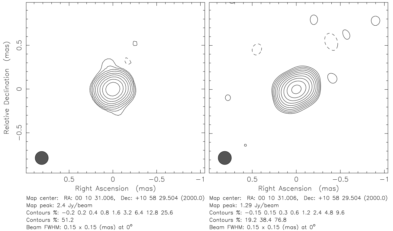
Abbildung 5.21: VLBA-Karte vom 14.09.1998 (links) und vom 12.12.1998 (rechts) von III Zw 2 bei 43 GHz rekonstruiert mit einem zirkularen 0.15 \times 0.15 mas Beam.
