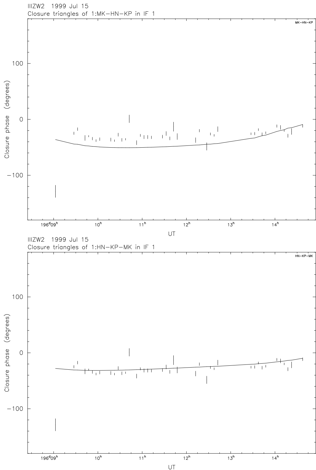
Abbildung 5.30: Wie in Abbildung 5.29. Bei der fünften Epoche reich jedoch selbst ein zweikomponentiges Modell (oben) nicht aus um die Daten zu erklären. Daher wurde bei dieser Epoche eine dritte Komponente hinzugefügt (unten).
