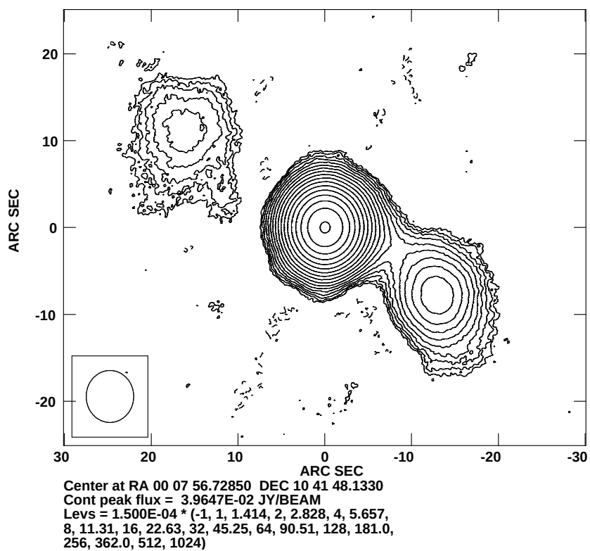
Abbildung 5.4: 4.8 GHz Karte von III Zw 2, zusammengesetzt aus 11 Epochen mit dem VLA in A, B, C und D-Konfiguration.
