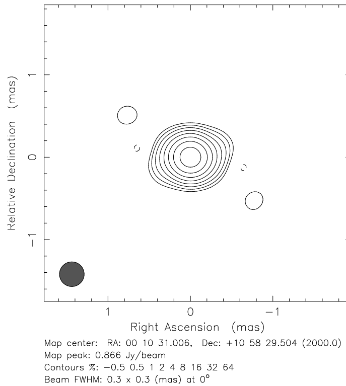
Abbildung 5.28: VLBA-Karte vom 15.07.1999 von III Zw 2 bei 15 GHz rekonstruiert mit einem zirkularen 0.3 \times 0.3 mas Beam.
